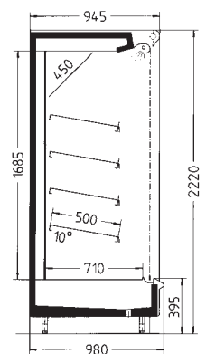
Methos 74.A4 L
