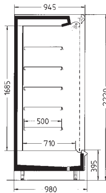
Methos 74.A3 L
