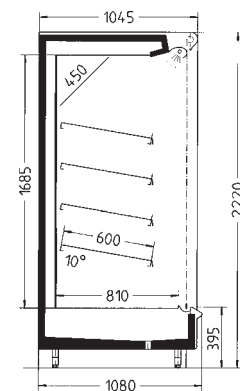
Methos 84.A4 L
