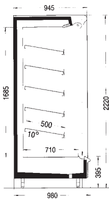
Methos 74.A5 L
