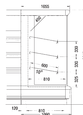
Methos 84.CE A4
