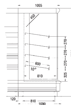
Methos 84.CE A4 L
