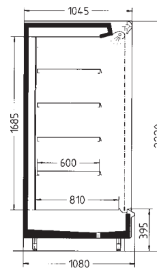
Methos 84.A3 L
