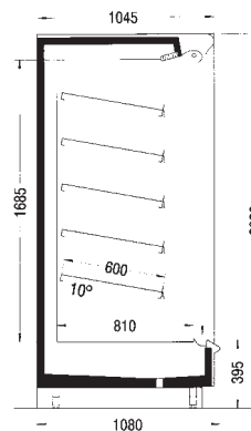
Methos 84.A5 L
